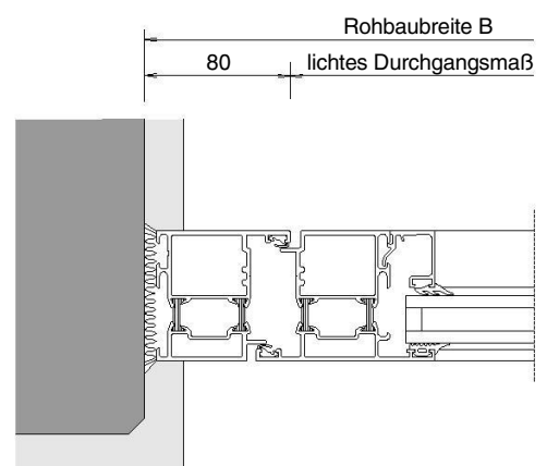
Stockprofil eingeputzt
