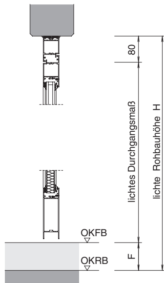
Türe ohne unterem Anschlag
