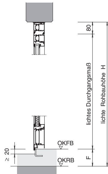
Türe mit unterem Anschlag
